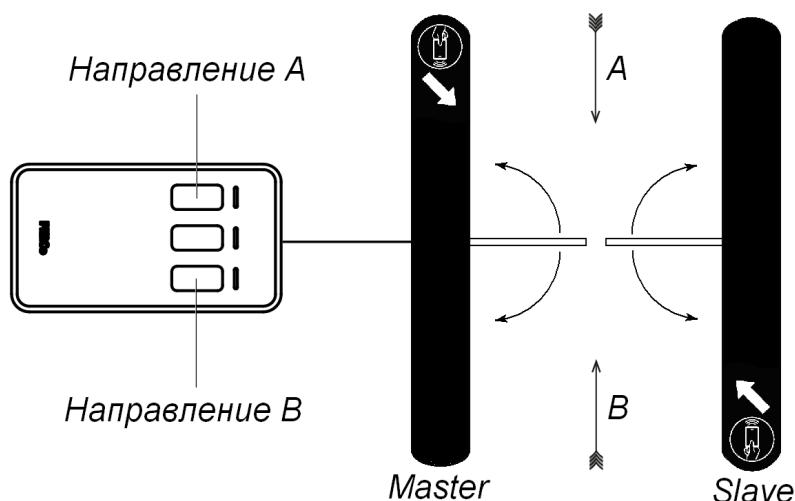
Рисунок 16. Стандартная ориентация ПДУ относительно секций турникета
