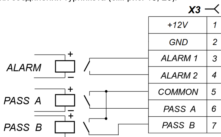
Рисунок 17. Выходные каскады для PASS A, PASS B и Alarm
