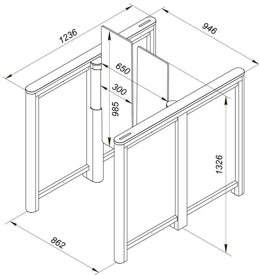
Рисунок 2. Габаритные размеры турникета со створками PERCo-ATG-300H
